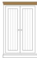
NEDBC30 H760 W660 D230 mm NEDBC31 H760 W660 D305 mm NEDBC32 H760 W660 D380 mm NEDBC33 H760 W965 D230 mm NEDBC34 H760 W965 D305 mm NEDBC35 H760 W965 D380 mm
